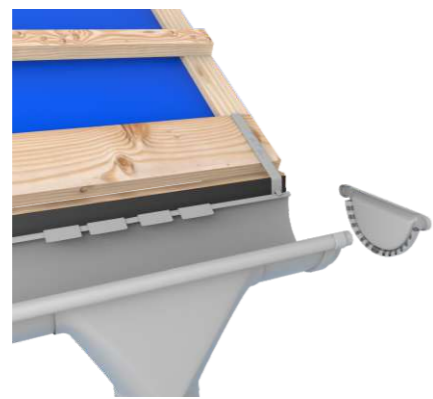
Denko montujemy po zamontowaniu rynny w uchwyty
